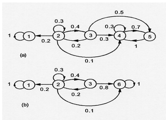
Figura 15: Clases comunicantes
