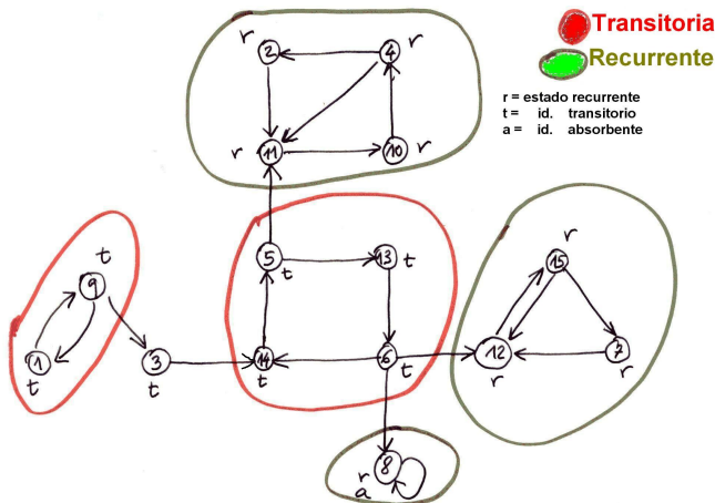
Figura 20: Cadena reducible.
