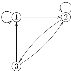
Figura 4: Digrafo fuertemente conexo.
