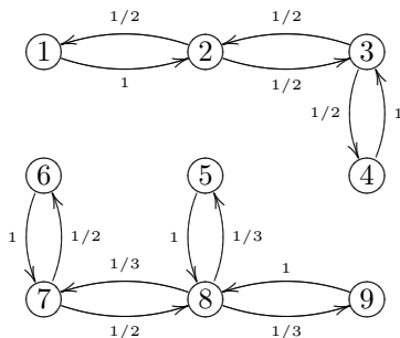
Figura 21: Digrafo ponderado del laberinto 3º.
