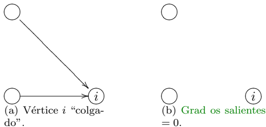
Figura 12: Vértices “colgados”.
