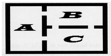
Figura 9: Laberinto 2º.
