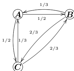
Figura 10: Digrafo ponderado del laberinto 2º.
