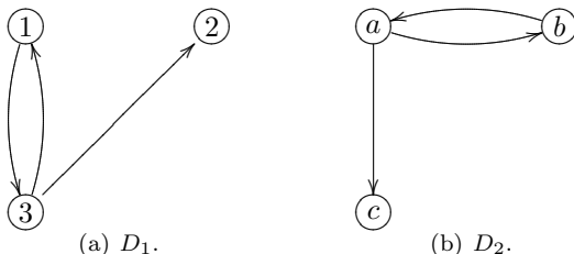
Figura 5: Digrafos isomorfos.
