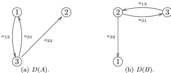
Figura 7: Digrafos \sigma -permutados.
