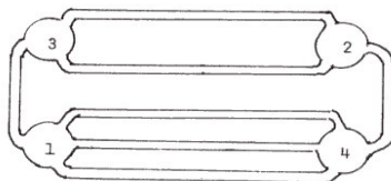
Figura 8: Laberinto 1º.
