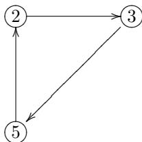
Figura 2: Ciclo C = (2, 3, 5, 2) .
